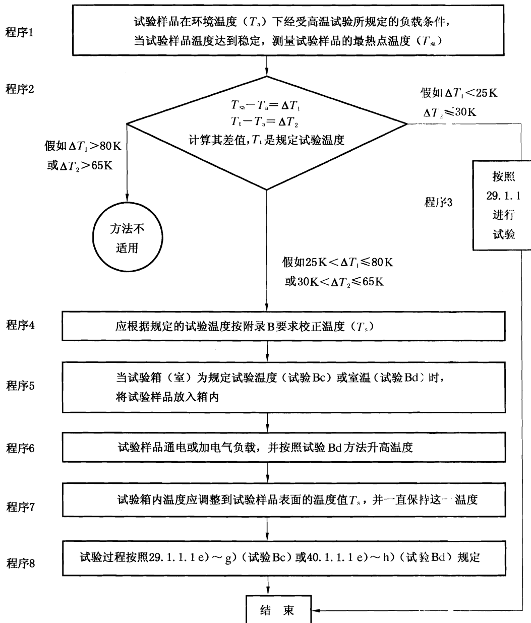
试验 Bc(29. 1. 2)和试验 Bd(40. 1. 2)中方法 B 简要流程图
