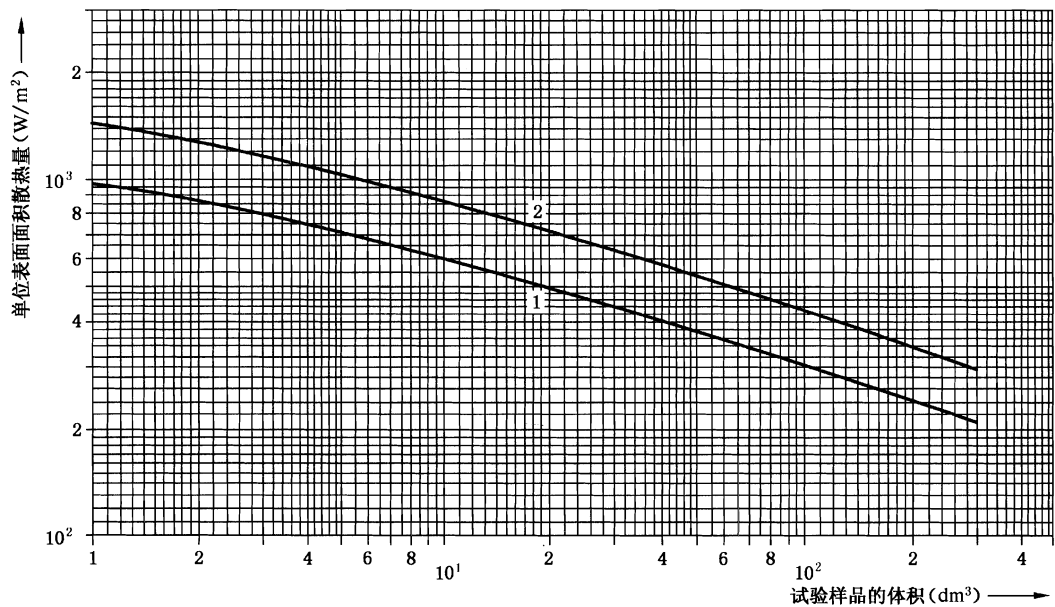
曲线 1 表示试验样品表面与箱壁之间距离为 10 cm 时,单位面积上允许的最大散热量与试验样品体积的关系; 曲线 2 表示当其距离为 20 cm 时两者的关系。
